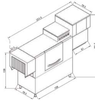
KONVEYÖRLÜ BULAŞIK YIKAMA MAKİNESİ 2000TBK/S
