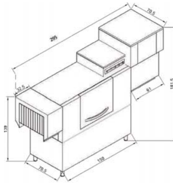
KONVEYÖRLÜ BULAŞIK YIKAMA MAKİNESİ 3000TBK/S
