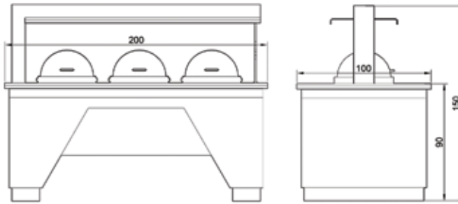
ÜÇLÜ ÇORBA ÜNİTESİ Ö. PERDELİ 2000X900X900X1500 TRIPLE SOUP STATION W. GLASS PROTECT 2000X900X900X1500
