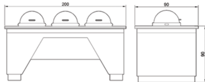
ÜÇLÜ ÇORBA ÜNİTESİ 200X90X90 TRIPLE SOUP STATION 200X90X90
